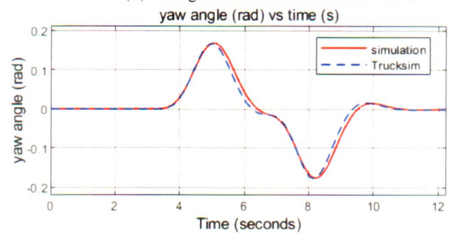
(d) Yaw angle for DLC
