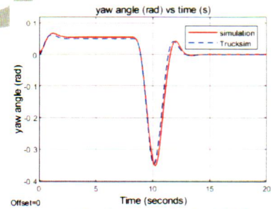
(d) Yaw angle for SLC
